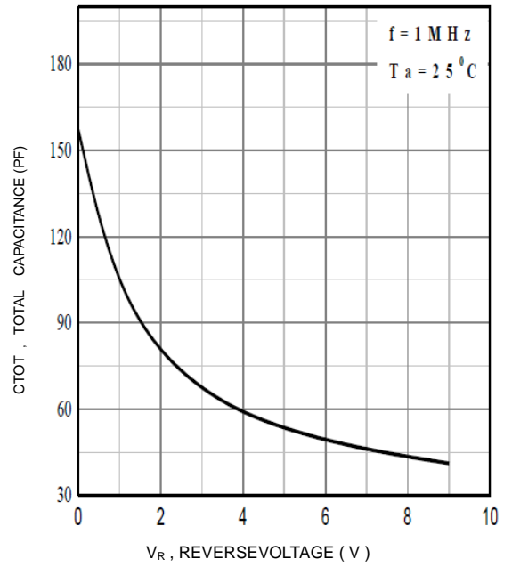
FIG-3 C_{TOT} -- V_R
