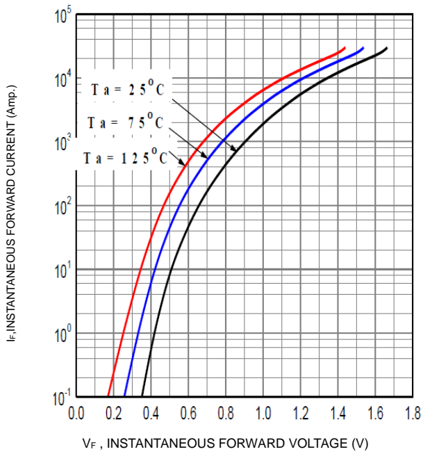
FIG-1 I_F — V_F
