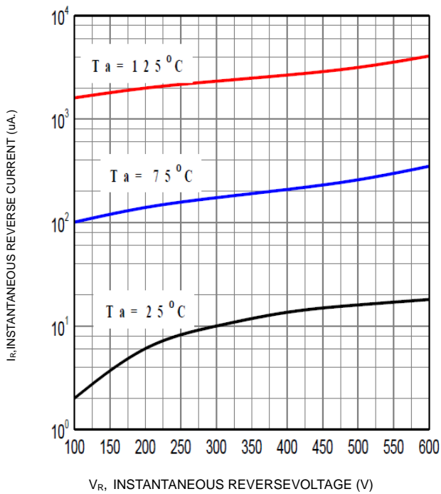
FIG-2 I_R — V_R
