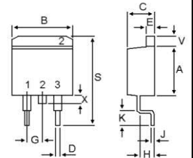
TO-263(D2-PAK)
