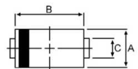
DO-214AC(SMA)
