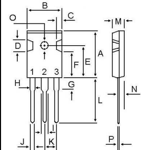
TO-247-3L
