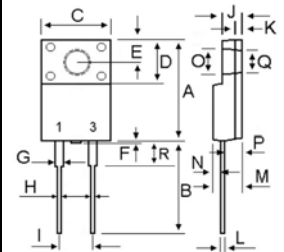
ITO-220A
