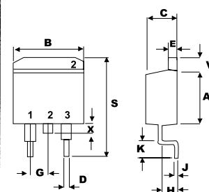
TO-263 (D2-PAK)
