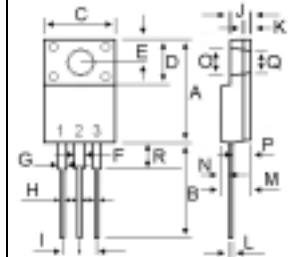
ITO-220AB
